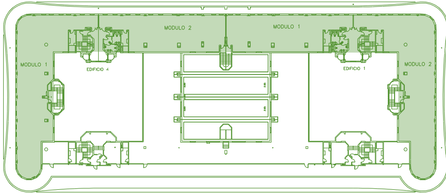
Planta 4
