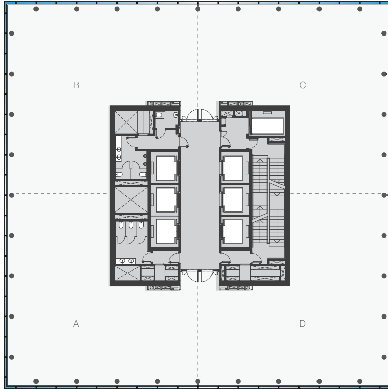
Planta Tipo 3-21
