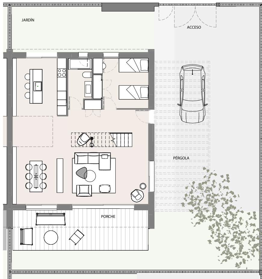
PLANTA BAJA
