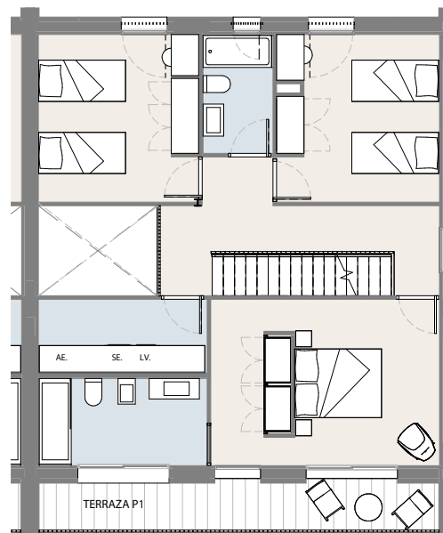
PLANTA PRIMERA
