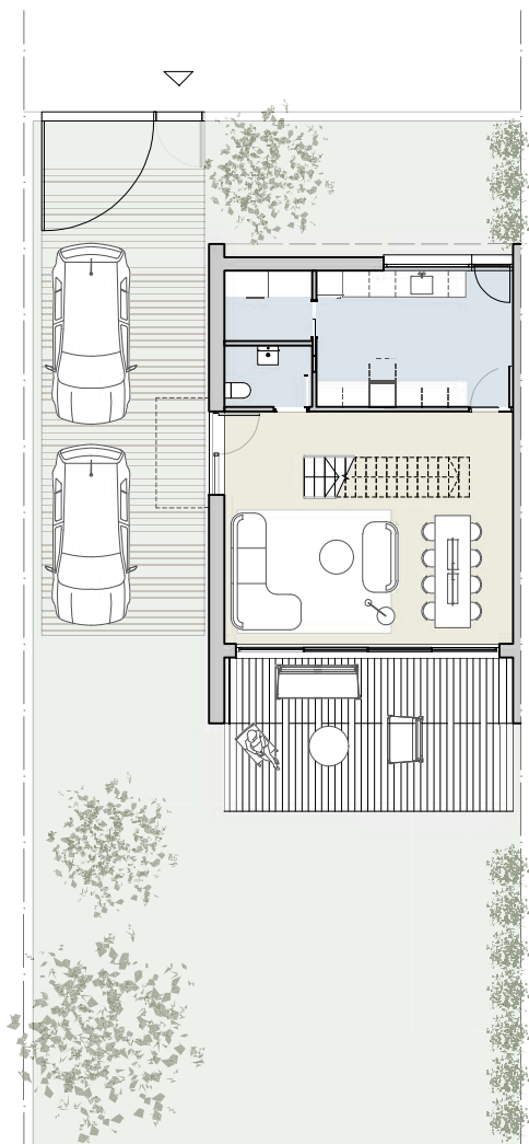
PLANTA BAJA
