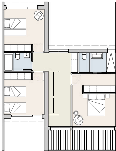
PLANTA PRIMERA
