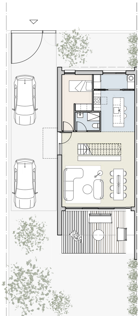
PLANTA BAJA
