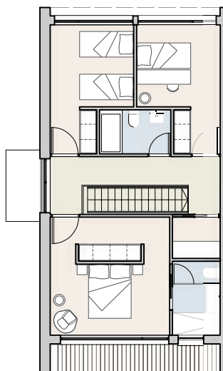
PLANTA PRIMERA
