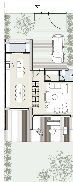
VIVIENDA TIPO 4
