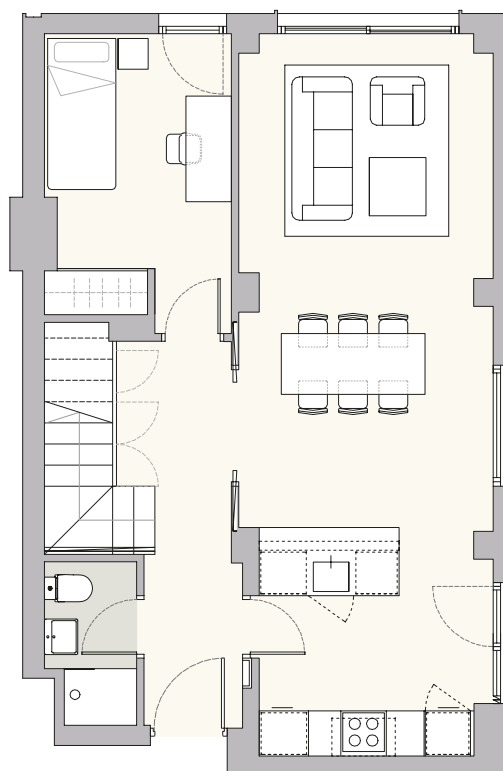
PLANTA BAJA
