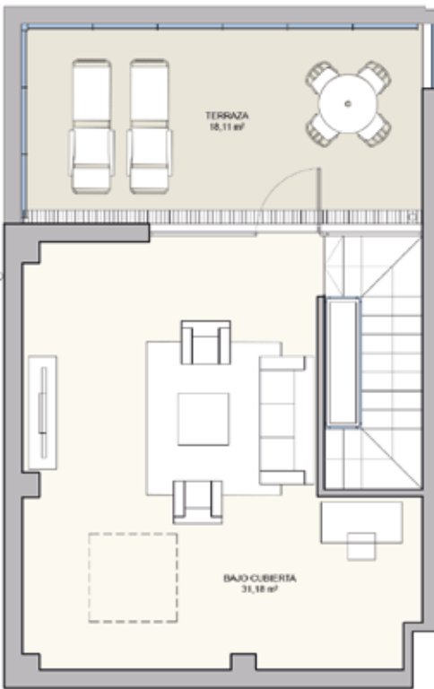
PLANTA BAJOCUBIERTA
