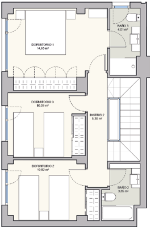
PLANTA PRIMERA
