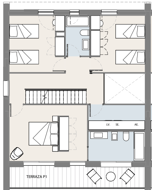
PLANTA PRIMERA
