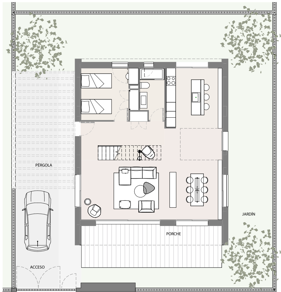
PLANTA BAJA
