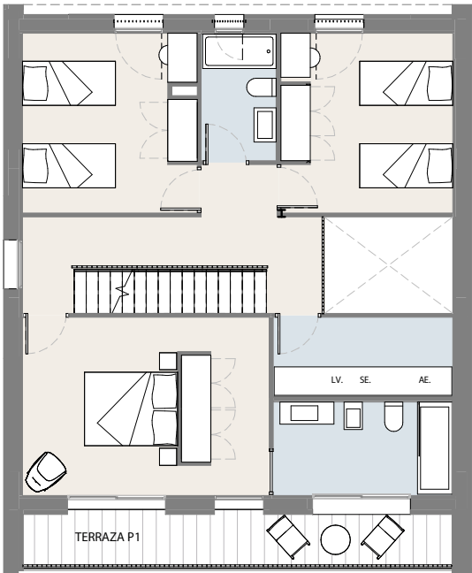
PLANTA PRIMERA
